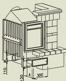
rúčka otočná - základná (RO)
